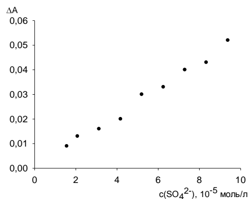
Рис. 6 Залежність поглинання іммобілізованого в желатиновій плівці комплексу Ва(II) з нітхромазо від концентрації \text{SO}_4^{2-} у водно-етанольному розчині при рН 1.5 і \lambda=675 нм.
