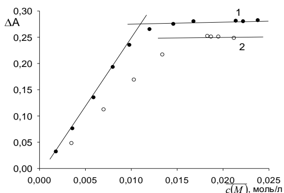
Рис. 3. Залежність поглинання іммобілізованих комплексів НРС з Fe(III) (1) при \lambda=720 нм і Cu(II) (2) при \lambda=495 нм від загальної концентрації металів в желатиновій плівці; \overline{c(R)}=0.03 моль/л.
